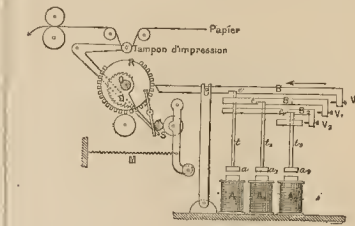
Fig. 2. Diseño del mecanismo del aparato receptor
